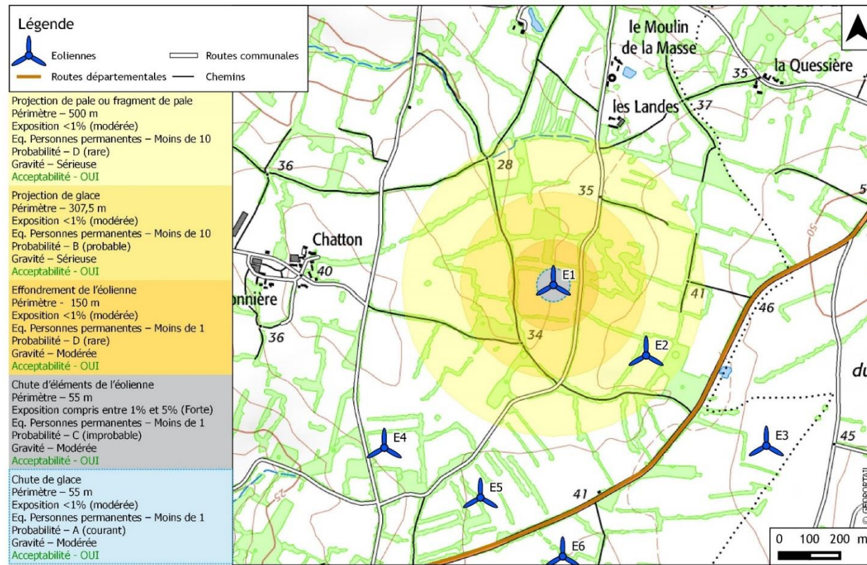
Synthèse des zones d'effet - éolienne E1 - VESTAS V110
