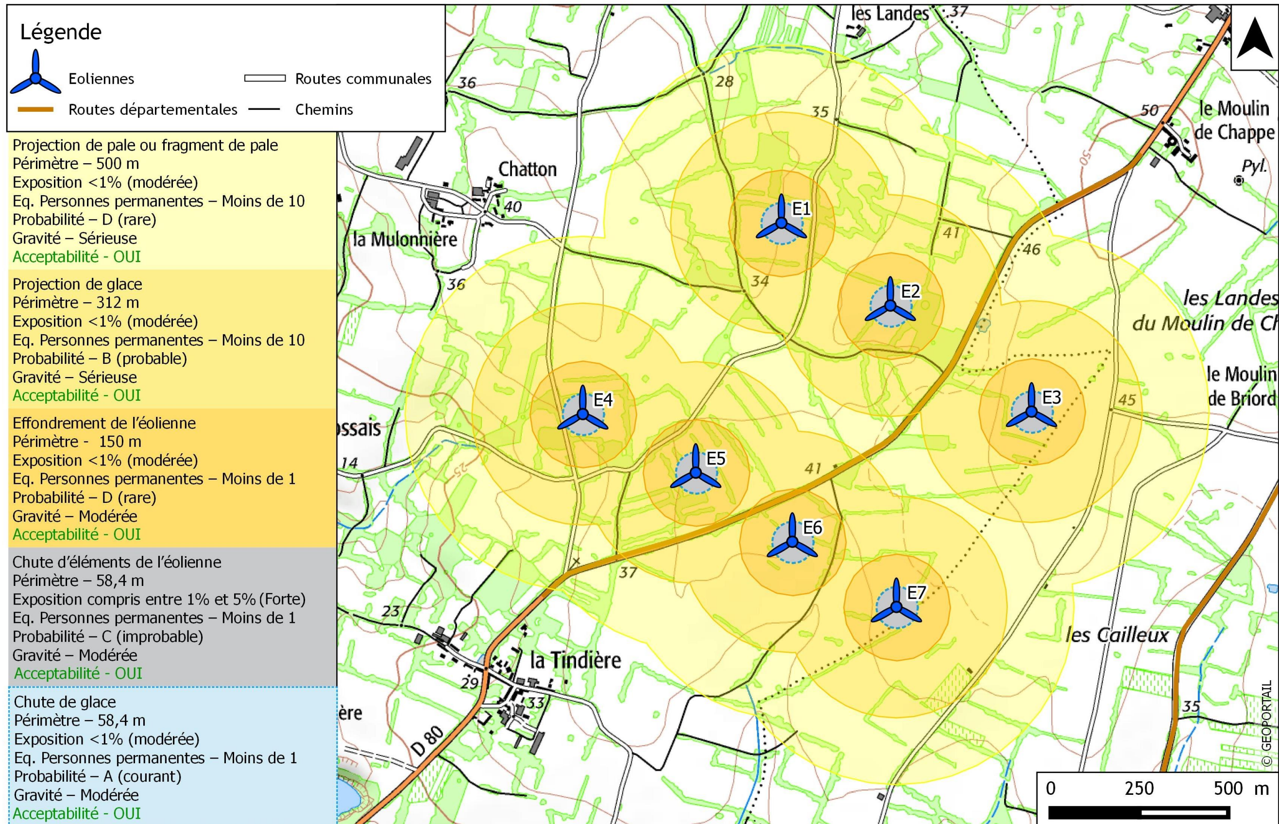
Cartographie de synthèse des risques - NORDEX N117
