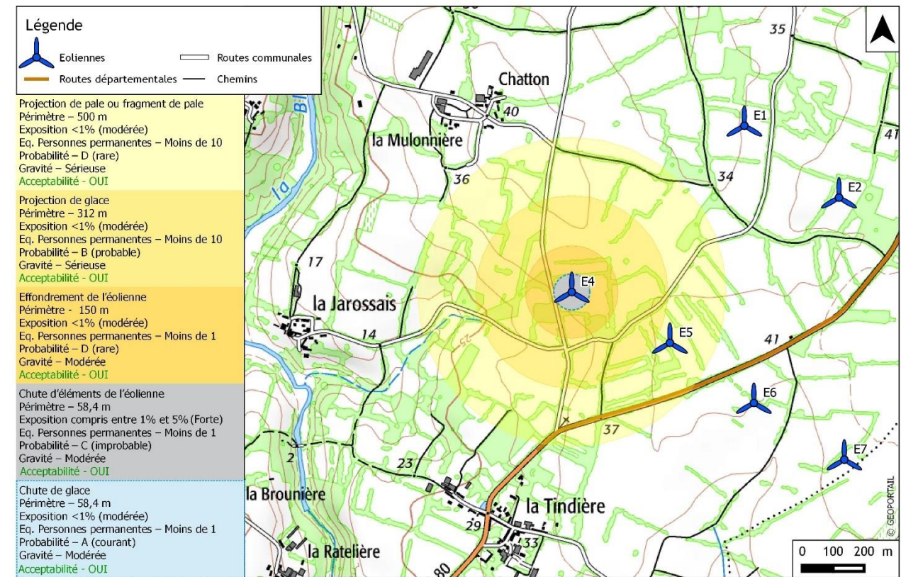
Synthèse des zones d'effet - éolienne E4 - NORDEX N117
