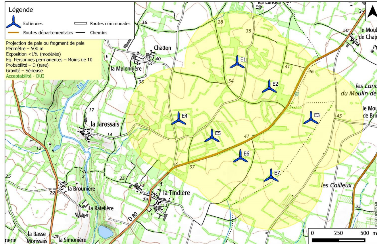
Zone d'effet du phénomène « Projection de pales ou de fragments de pales » - VESTAS V110 et NORDEX N117
