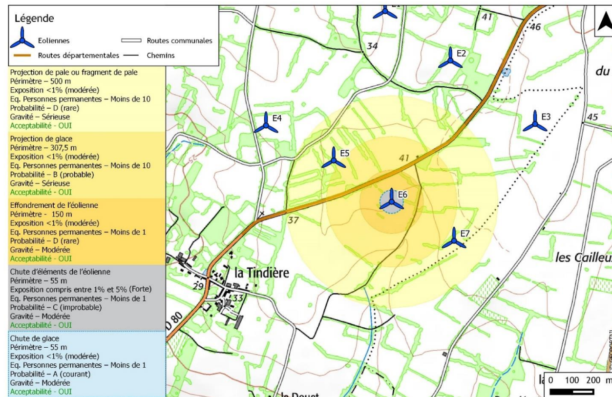
Synthèse des zones d'effet - éolienne E6 - VESTAS V110
