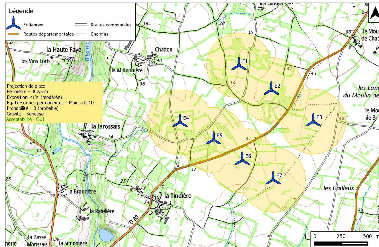
Zone d'effet du phénomène « Projection de glace » - VESTAS V110
