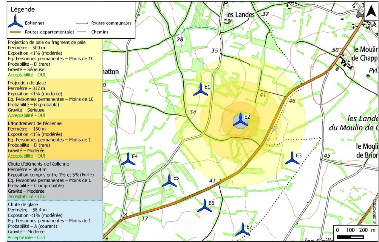
Synthèse des zones d'effet - éolienne E3 - NORDEX N117
