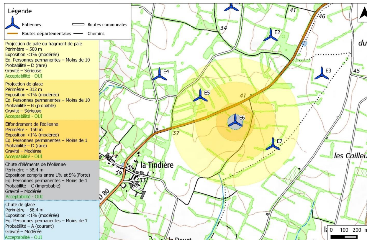
Synthèse des zones d'effet - éolienne E6 - NORDEX N117
