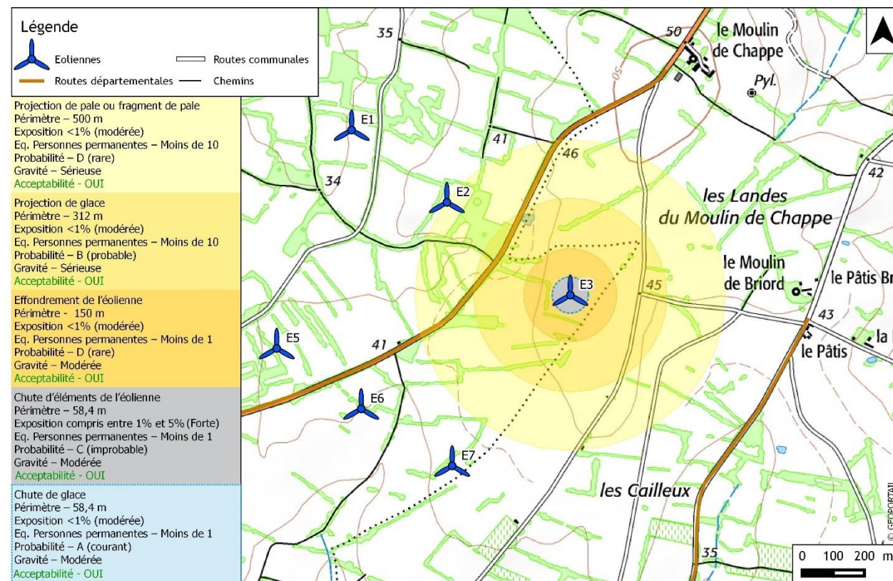
Synthèse des zones d'effet - éolienne E2 - NORDEX N117
