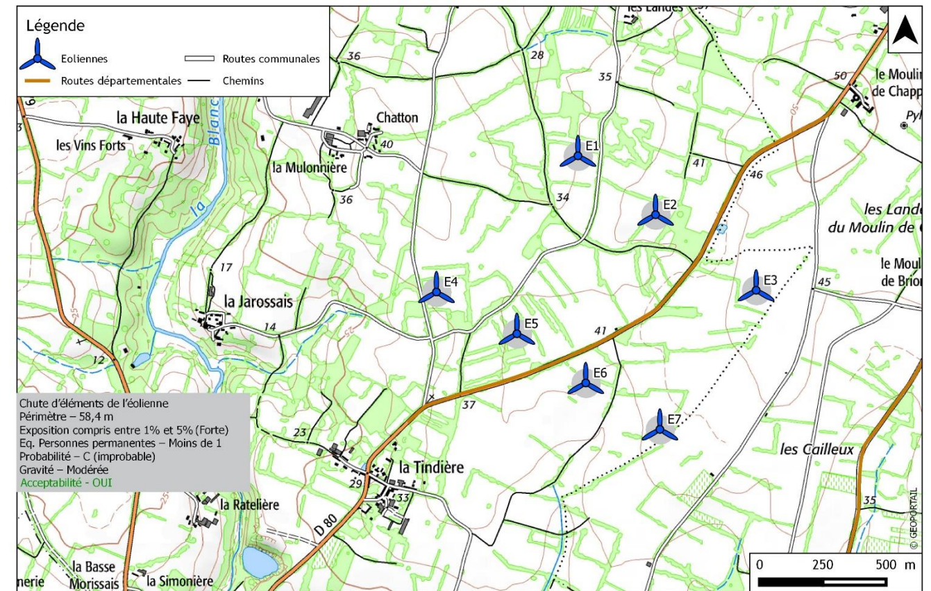
Zone d'effet du phénomène « Chute d'éléments de l'éolienne » - NORDEX N117
