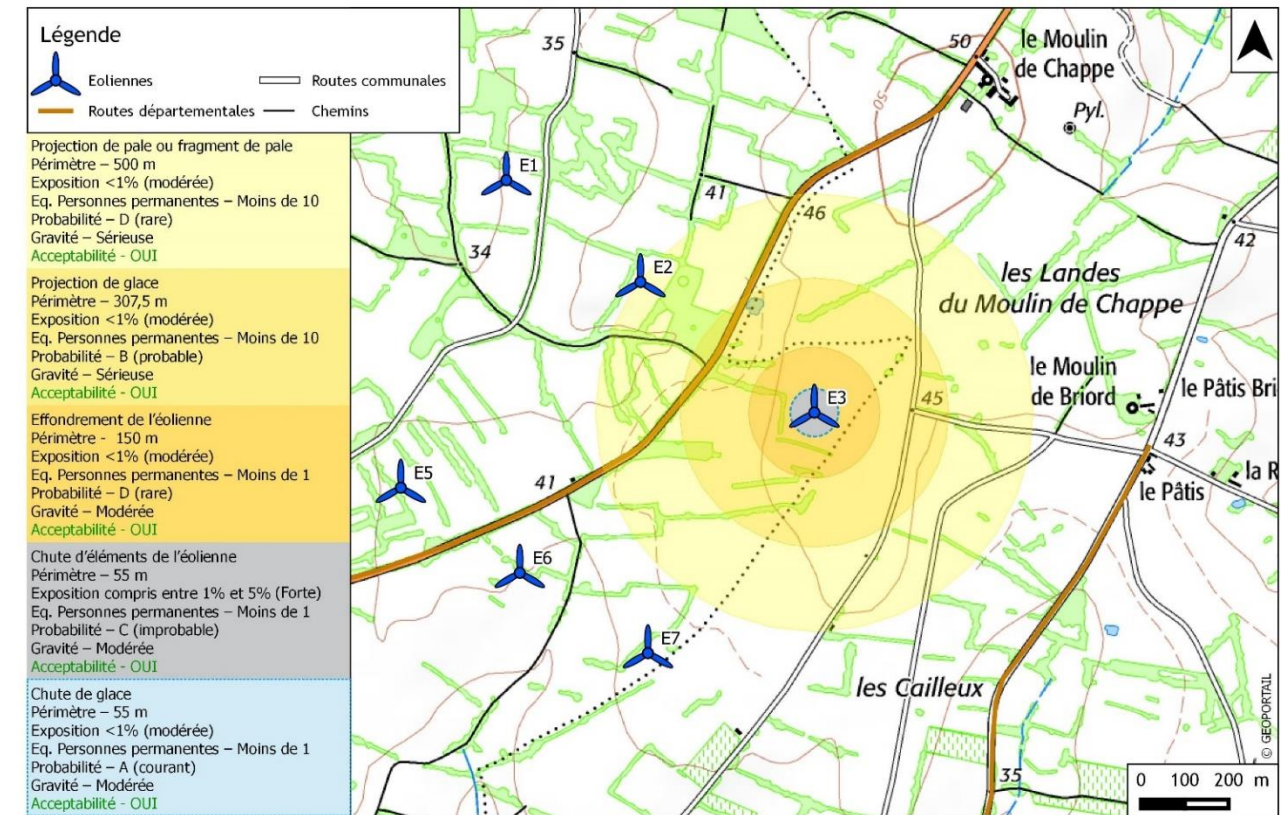
Synthèse des zones d'effet - éolienne E3 - VESTAS V110
