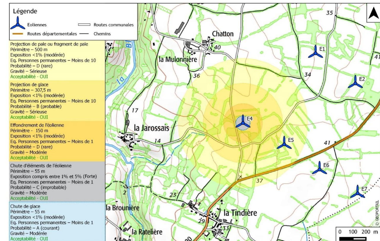
Synthèse des zones d'effet - éolienne E4 - VESTAS V110
