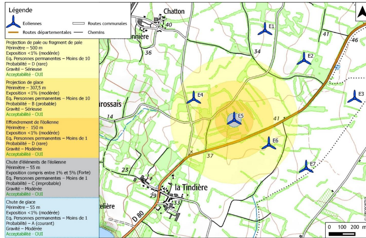
Synthèse des zones d'effet - éolienne E5 - VESTAS V110
