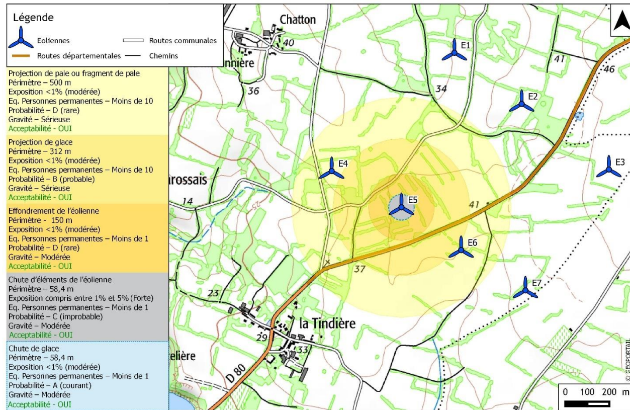
Synthèse des zones d'effet - éolienne E5 - NORDEX N117
