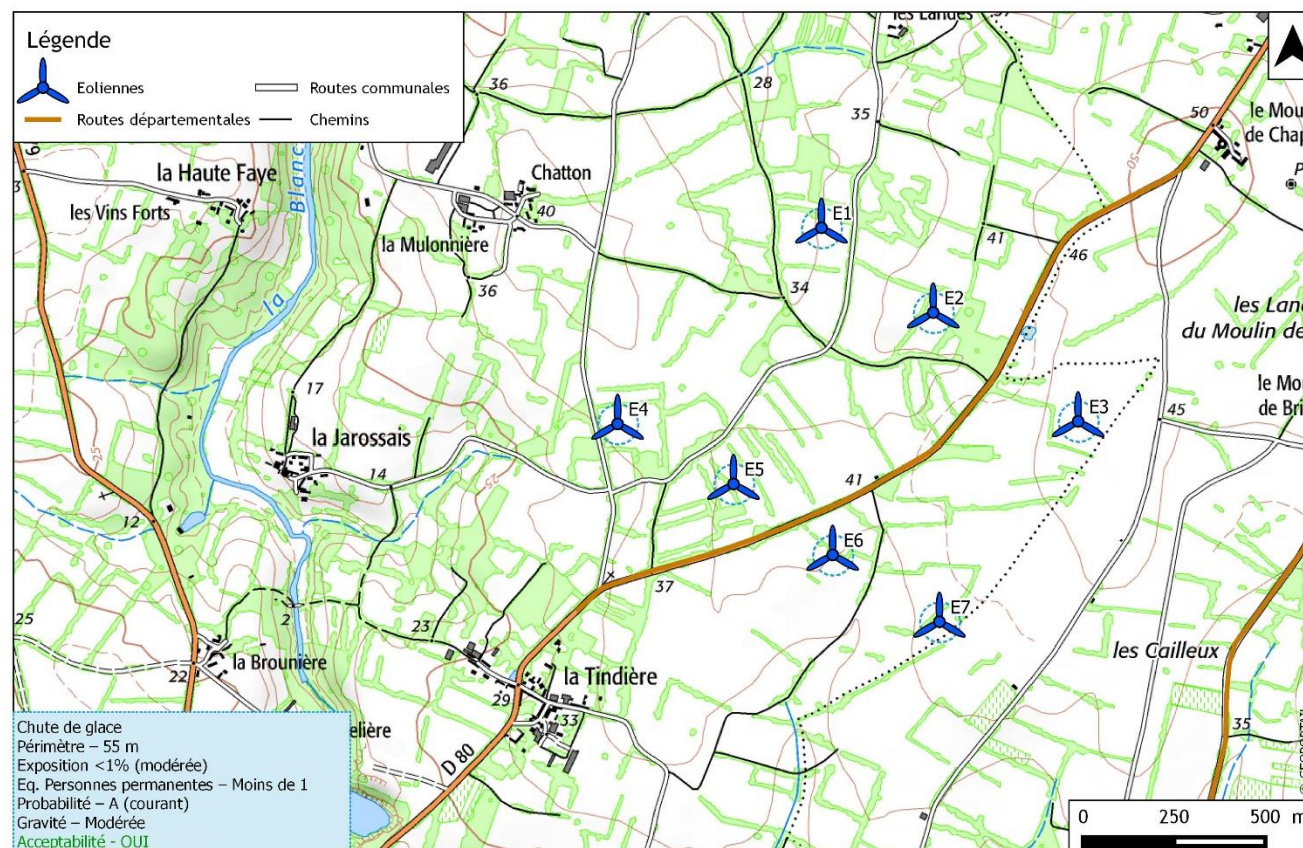
Zone d'effet du phénomène « Chute de glace » - VESTAS V110
