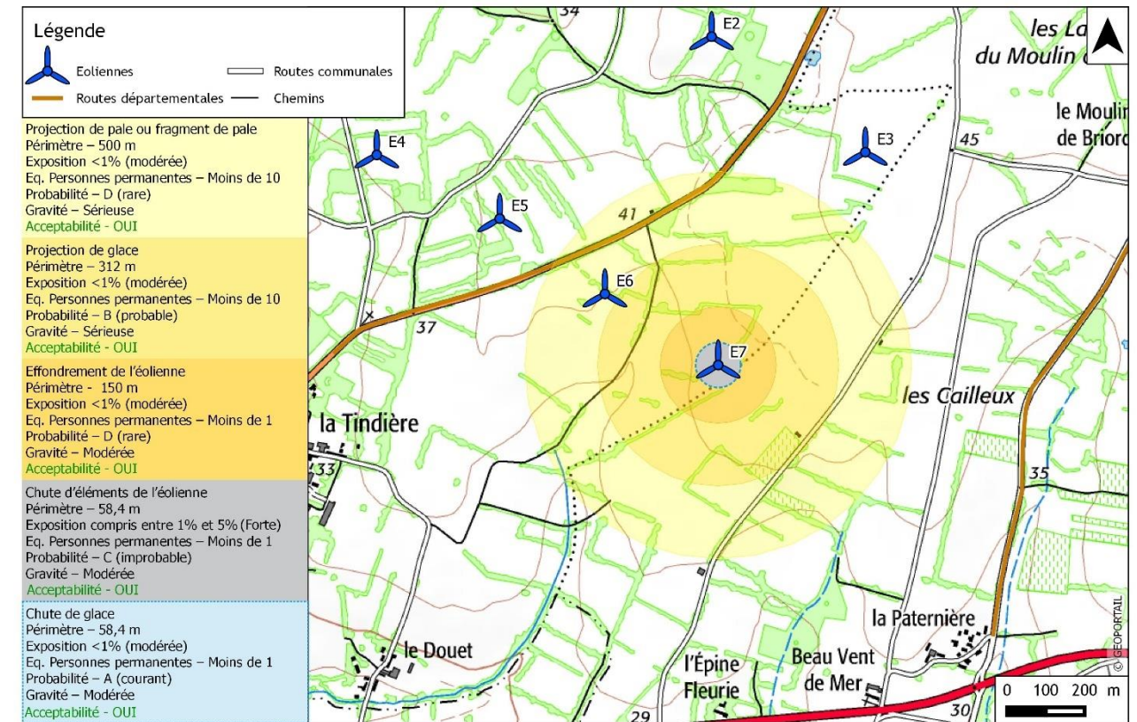
Synthèse des zones d'effet - éolienne E7 - NORDEX N117
