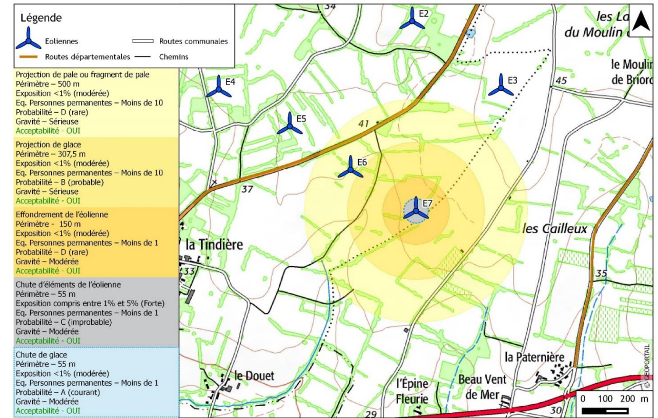
Synthèse des zones d'effet - éolienne E7 - VESTAS V110
