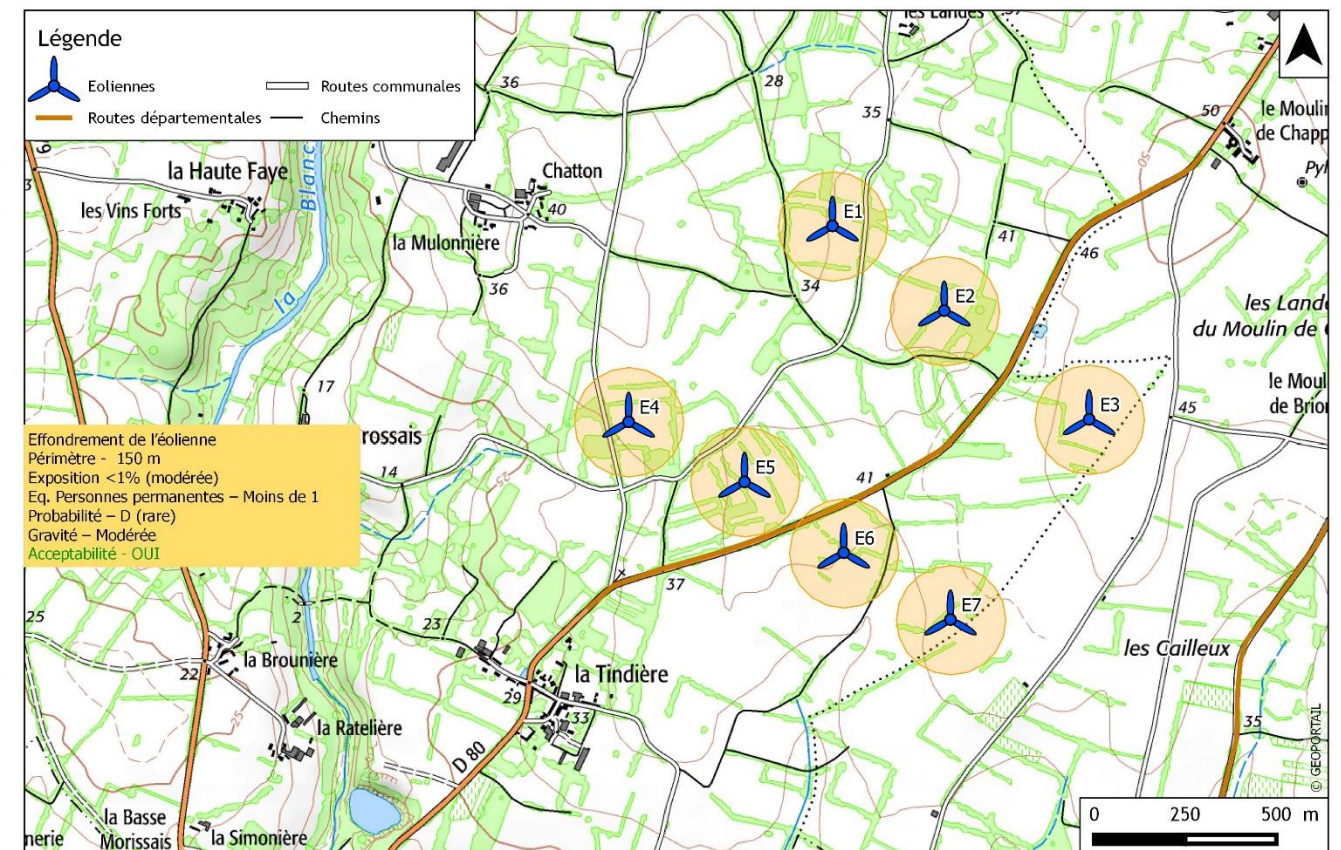
Zone d'effet du phénomène « Effondrement de l'éolienne » - NORDEX N117
