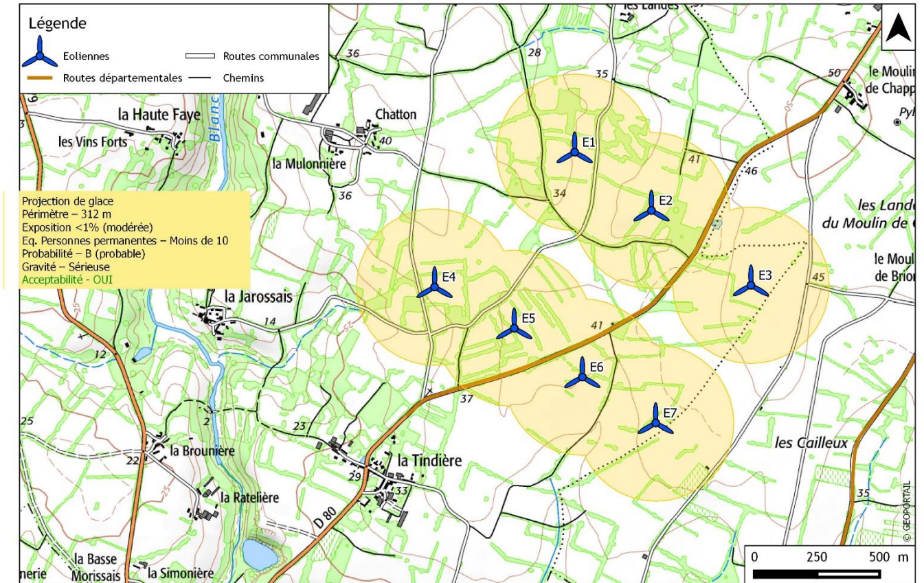
Zone d'effet du phénomène « Projection de glace » - NORDEX N117
