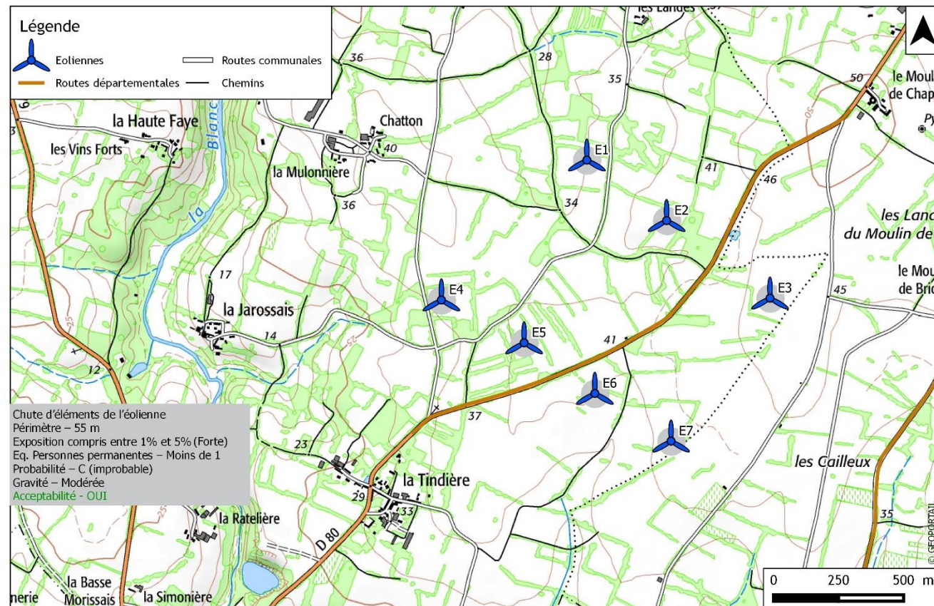
Zone d'effet du phénomène « Chute d'éléments de l'éolienne » - VESTAS V110
