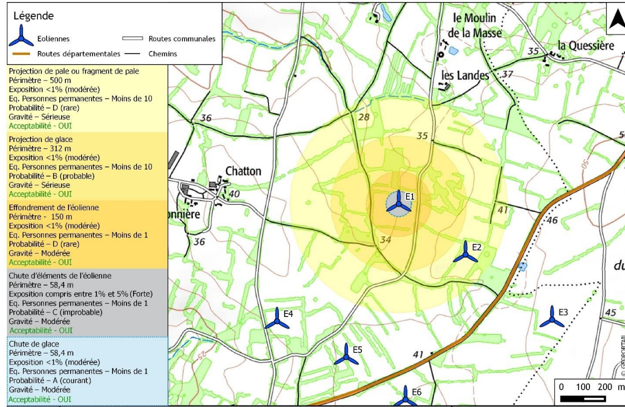
Synthèse des zones d'effet - éolienne E1 - NORDEX N117
