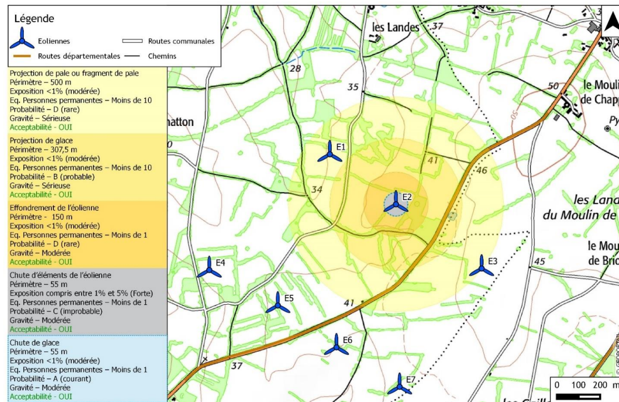
Synthèse des zones d'effet - éolienne E2 - VESTAS V110
