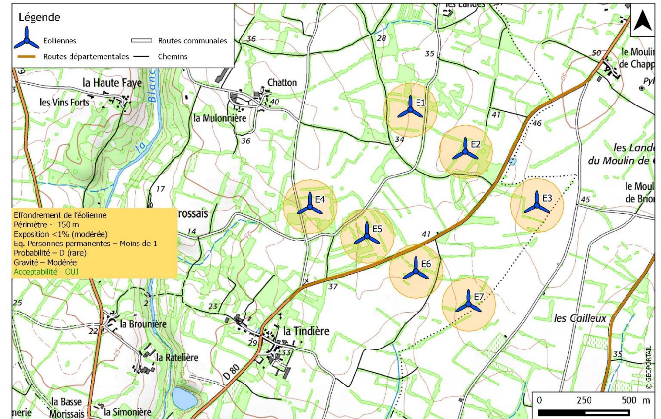
Zone d'effet du phénomène « Effondrement de l'éolienne » - VESTAS V110
