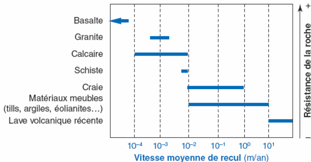
Recul moyen des falaises en fonction des matériaux constitutants (Woodroffe, 2002)
