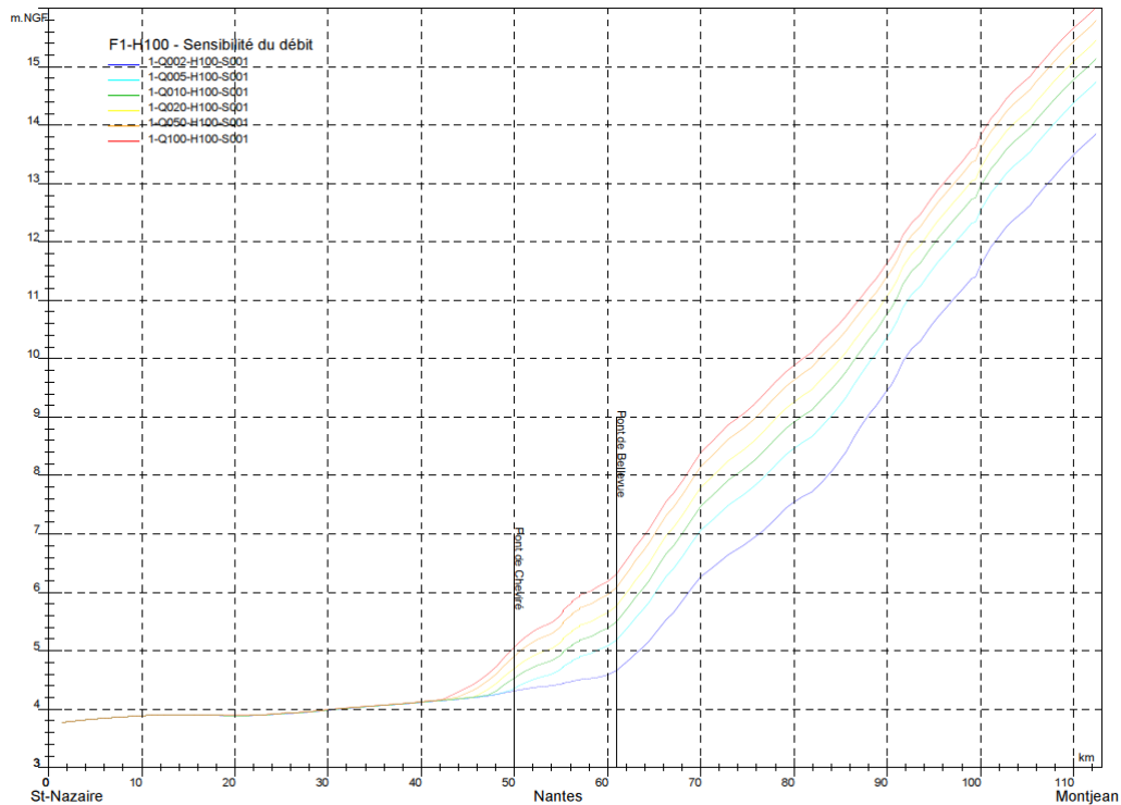
Fig. 5. NIVEAUX D'EAU MAXIMAUX POUR DIFFÉRENTS DÉBITS DE LA LOIRE AVEC UN NIVEAU AVAL CENTENNAL (SOURCE : « LIGNES D'EAU DE CRUES DANS L'ESTUAIRE DE LA LOIRE » RÉALISÉE POUR LE GIP LOIRE ESTUAIRE)
