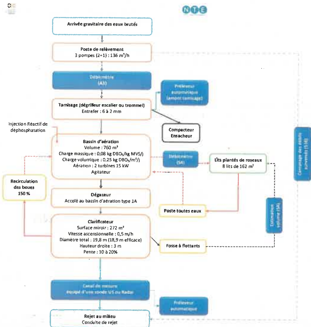
Figure 46 - Synoptique simplifié de la future station d'épuration
